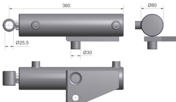
Figuur 3.2.3-Side-shift cilinder 70-30-200 (O.M)
