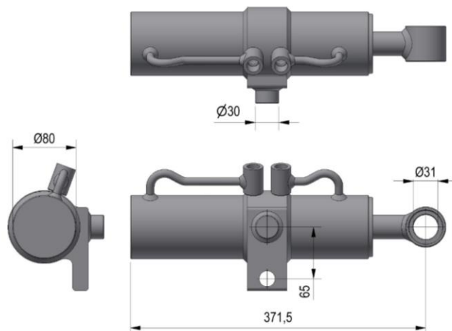
Figuur 4.2.3-Side-shift cilinder 70-30-200 Rechts
