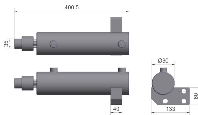
Figuur 5.1.3-Cilinder DW 70-30-200 t.b.v. rechtsdraaiend
