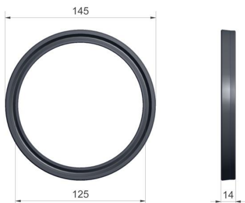
Figuur 3.3.10-Manchet Ø145x125-L14 H9
