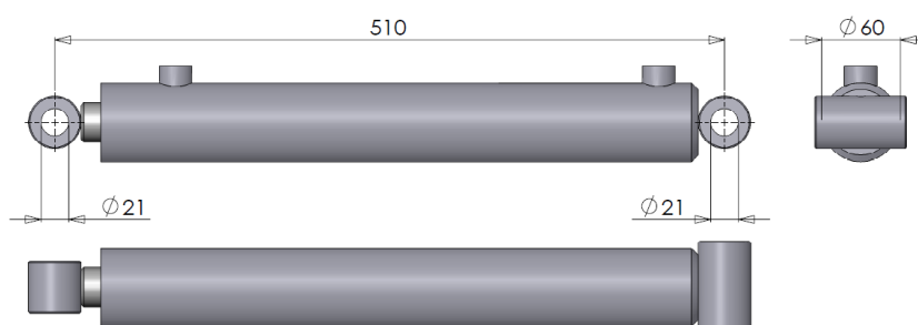
Figuur 9.1.1-Cilinder DW 50-30-330
