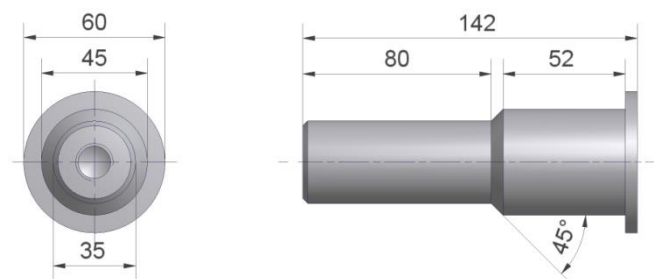
Figuur 12.2-Draaipen Ø45/35-L142 (Art. nr. 429080)
