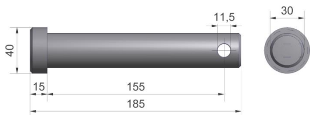
Figuur 12.3-Pen klemplaat Ø30-L170 (Art. nr. 4290771)
