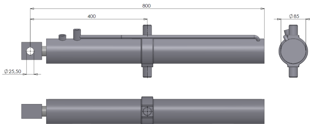
Figuur 2.2.9-Cilinder DW 70-35-600
