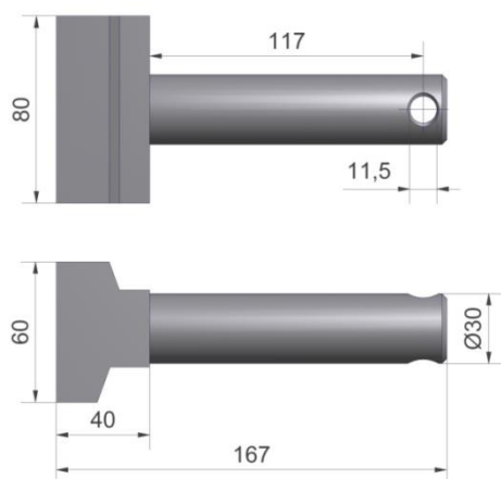
Figuur 12.5-Klemplaat inc. pen FEM II/III (Oud) (Art. nr. 4290095)
