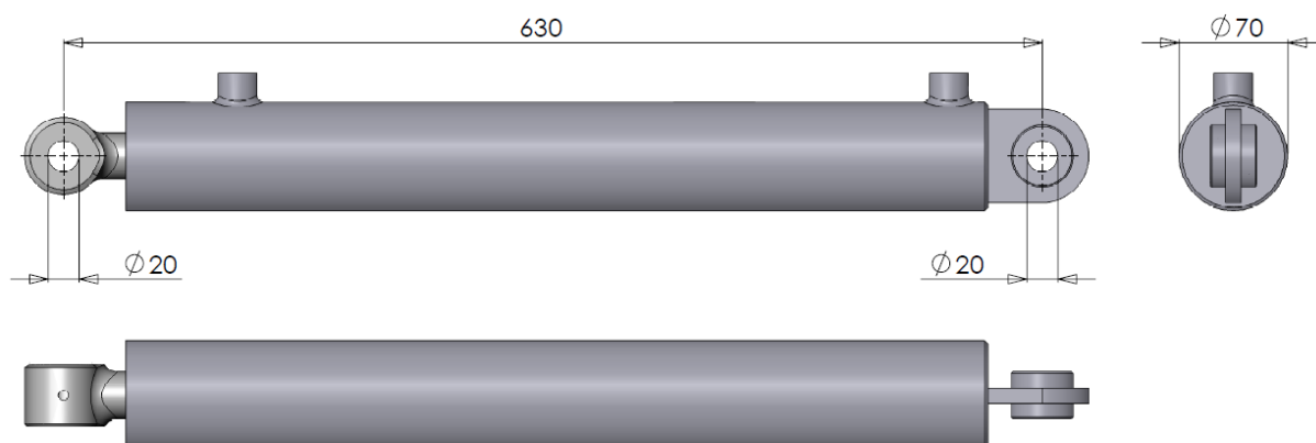
Figuur 7.1.1-Cilinder DW 60-30-410
