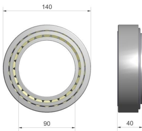
Figuur 5.2.1-Kegellager 33018
