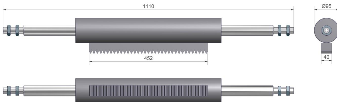
Figuur 3.1.6-Cilinder DW 80-40-377 (oud model)
