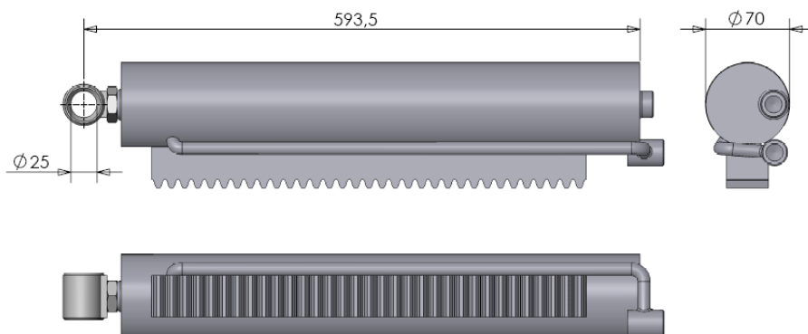
Figuur 3.1.5-Cilinder DW 60-30-420 t.b.v. draaislag 200° (oud model)
