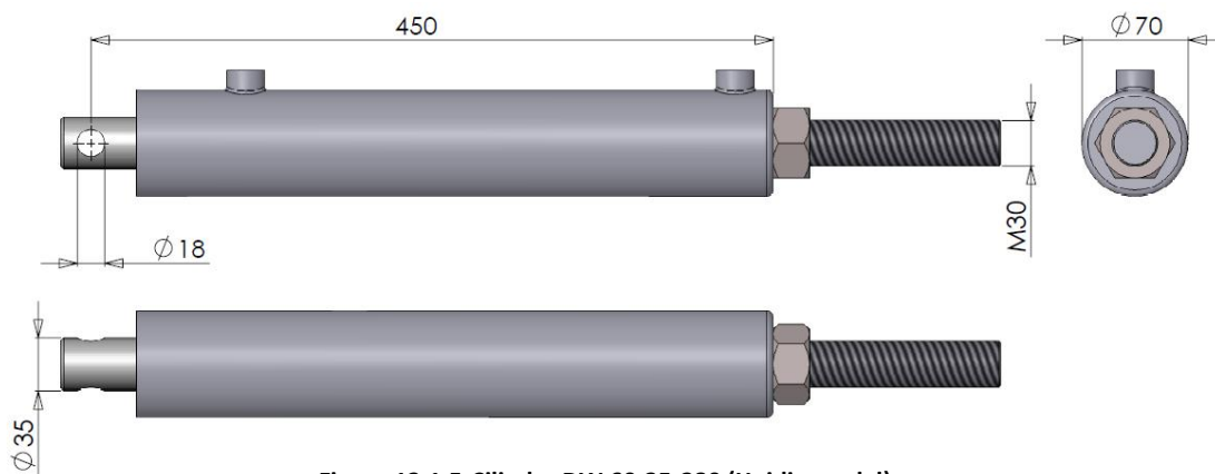
Figuur 12.1.5-Cilinder DW 60-35-280 (Huidig model)
