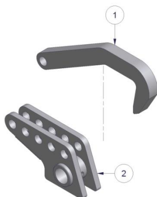
Figuur 2.1.2-Borghaak nieuw model
