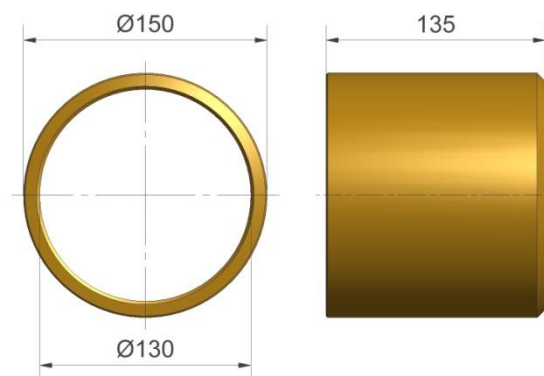
Figuur 3.3.5-Bronzen bus 150x130-L135
