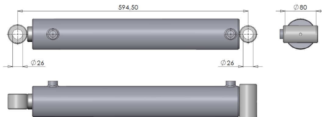
Figuur 12.1.1-Cilinder DW 70-40-410
