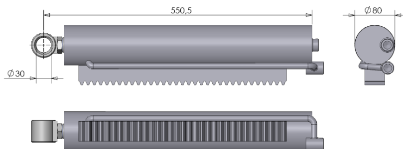
Figuur 3.1.2-Cilinder DW 70-30-377 t.b.v. draaislag 180° (oud model)
