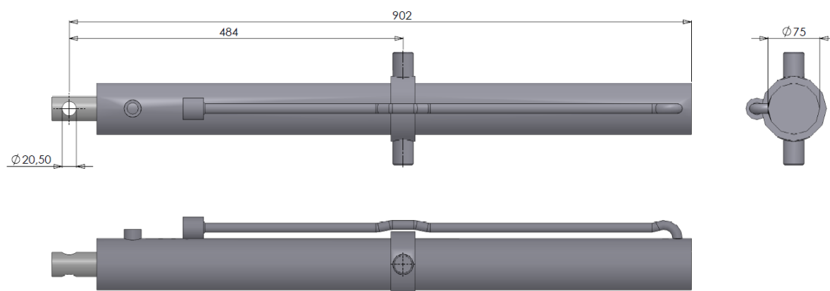
Figuur 2.2.3-Cilinder DW 63-35-750
