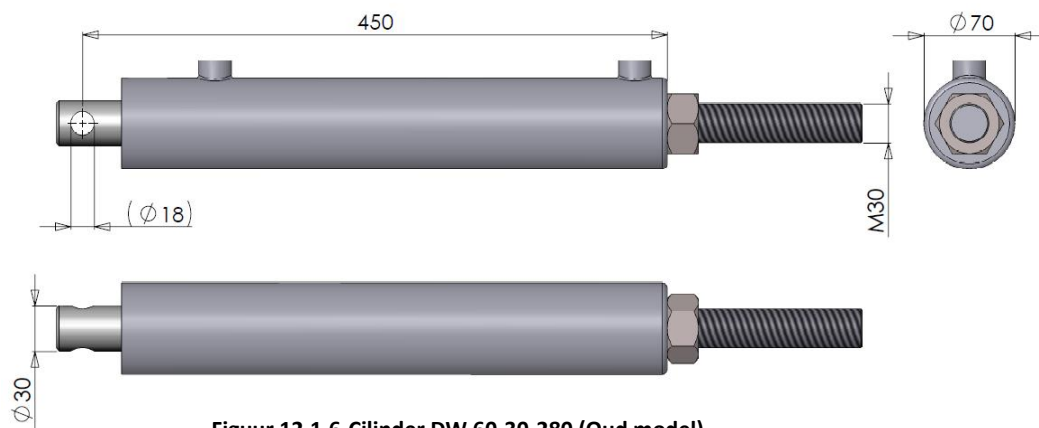
Figuur 12.1.6-Cilinder DW 60-30-280 (Oud model)
