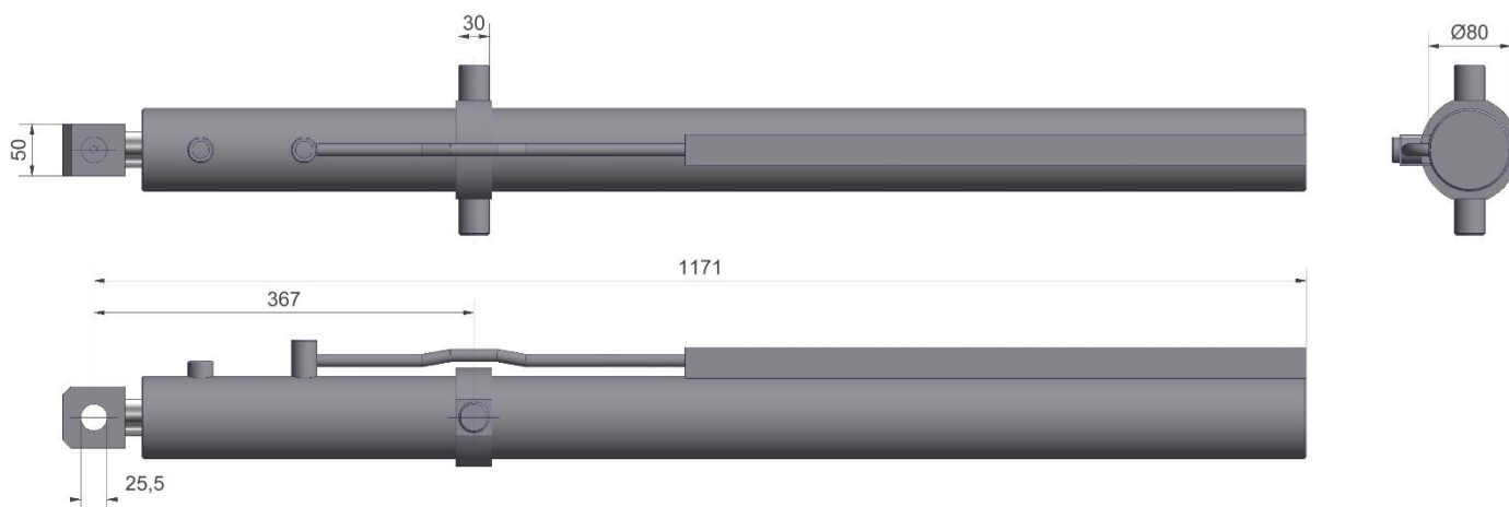
Figuur 2.2.6-Cilinder DW 70-35-1000 Blok
