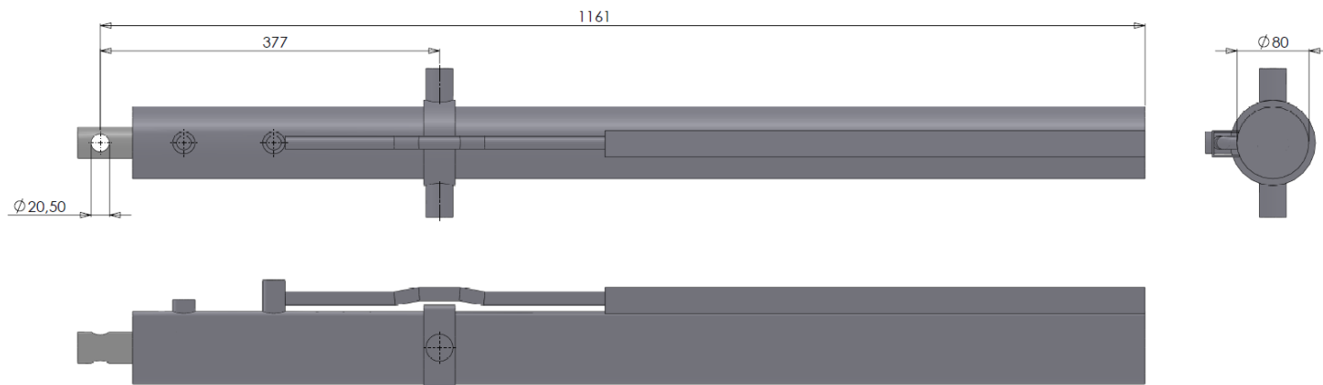
Figuur 2.2.5-Cilinder DW 70-35-1000
