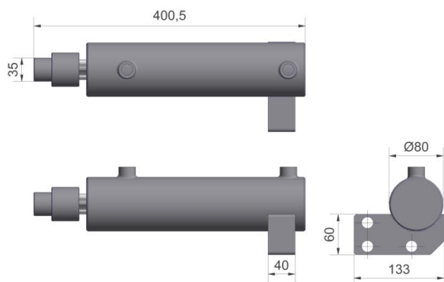
Figuur 5.1.2-Cilinder DW 70-30-200 t.b.v. linksdraaiend
