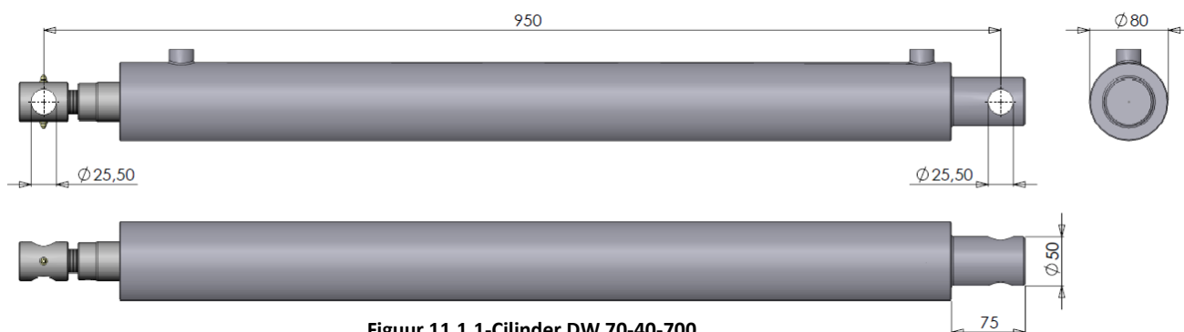
Figuur 11.1.1-Cilinder DW 70-40-700
