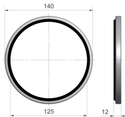
Figuur 3.3.7-Afstrijker 125x140x9/12
