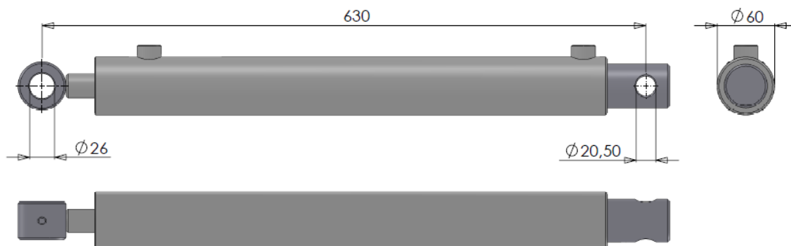
Figuur 12.1.9-Cilinder DW 50-25-410 (Oud model)
