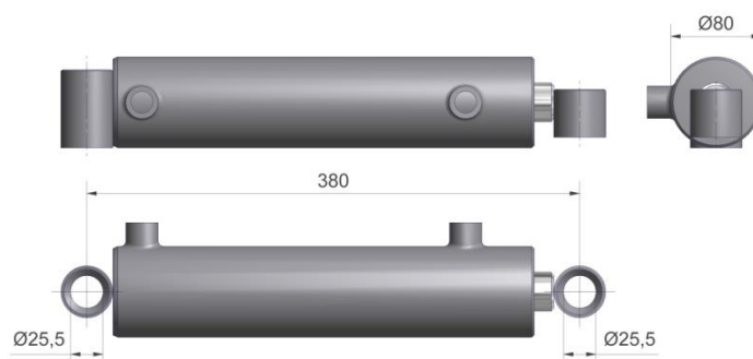
Figuur 3.2.5-Side-shift cilinder 70-30-200
