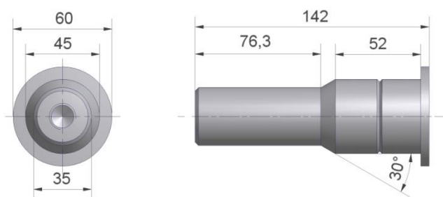
Figuur 12.1-Draaipen Ø45/35-L142 (Art. nr. 4290797)
