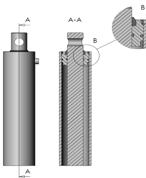
Figuur 2.2.2-Cilinder uitgevoerd met een gladde kop (GK)
