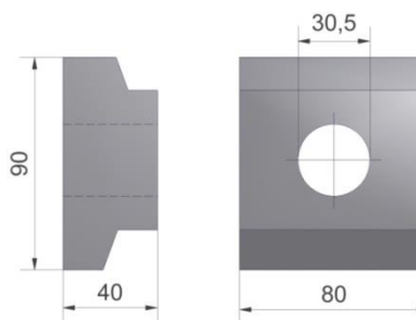
Figuur 12.4-Klemplaat los FEM II/III (Art. nr. 4290094)
