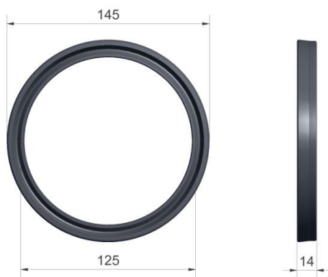
Figuur 5.2.3-Manchet Ø145x125-L14 H9
