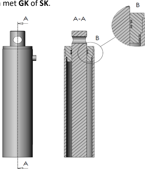
Figuur 2.2.1-Cilinder uitgevoerd met een schroefbare kop (SK)
