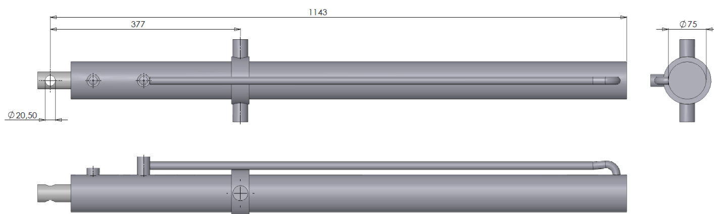
Figuur 2.2.4-Cilinder DW 63-35-1000
