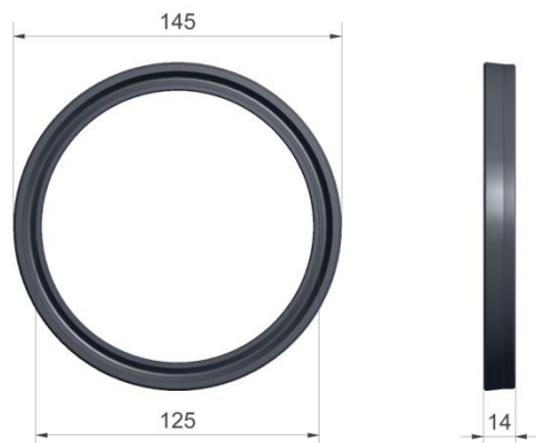
Figuur 4.3.5-Manchet Ø145x125-L14 H9
