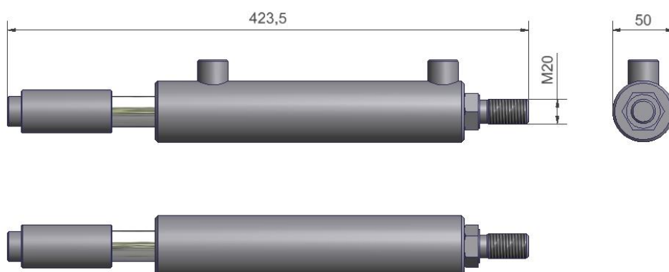
Figuur 11.1.3-Cilinder DW 40-25-150
