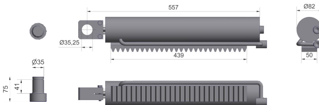
Figuur 4.1.1-Cilinder DW 70-30-377 M5 t.b.v. draaislag 180°
