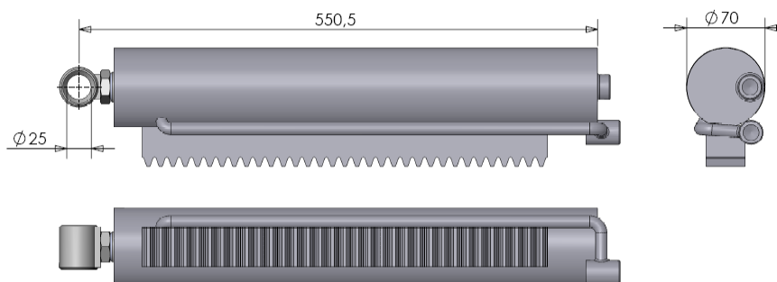
Figuur 3.1.3-Cilinder DW 60-30-377 t.b.v. draaislag 180° (oud model)
