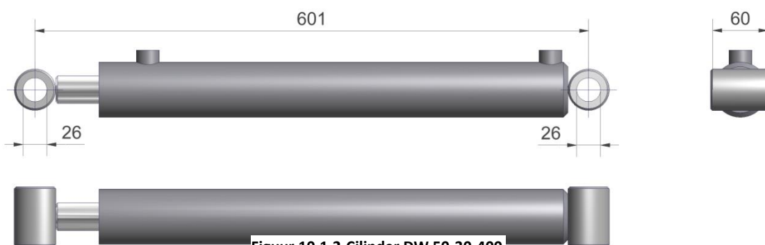
Figuur 10.1.2-Cilinder DW 50-30-400
