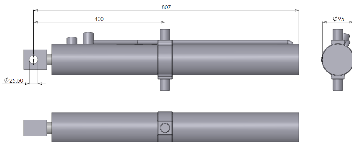
Figuur 2.2.8-Cilinder DW 80-35-600
