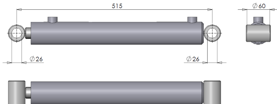
Figuur 12.1.4-Cilinder DW 50-30-330
