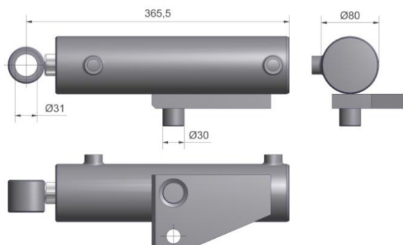
Figuur 4.2.1-Side-shift cilinder 70-30-200
