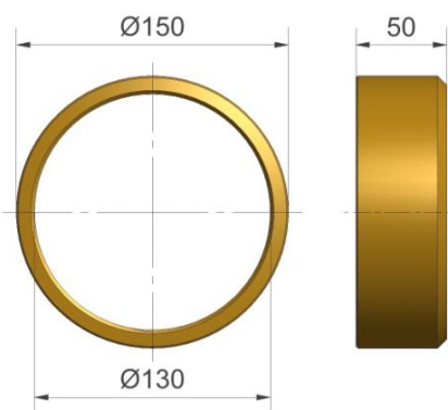
Figuur 3.3.3-Bronzen bus 150x130-L50
