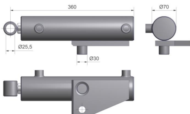
Figuur 3.2.1-Side-shift cilinder 60-30-200
