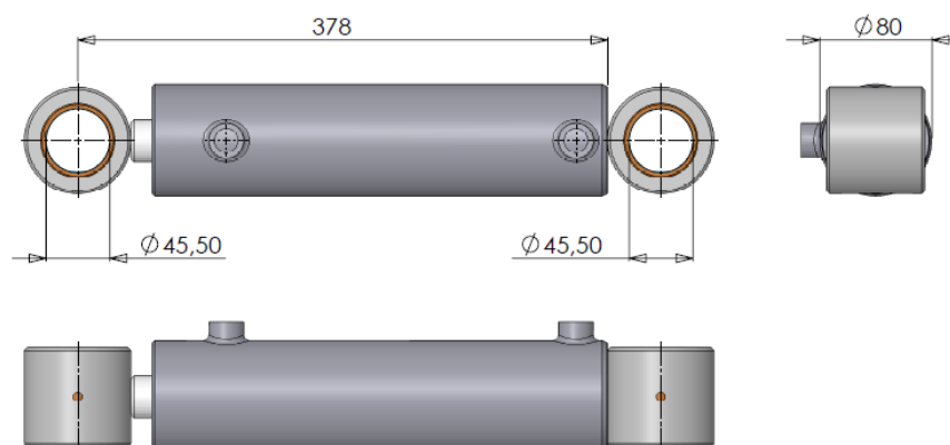
Figuur 2.2.7-Cilinder DW 70-30-200
