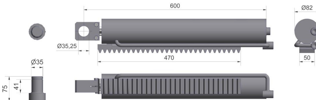
Figuur 4.1.2-Cilinder DW 70-30-377 M5 t.b.v. draaislag 200°
