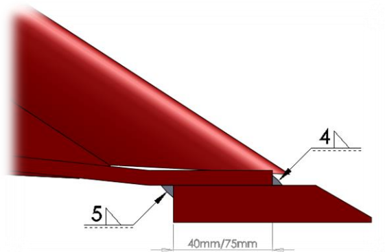
Abbildung 3.6.1 - Überlappungsschaufel für hydraulische Streifen abnutzen:
