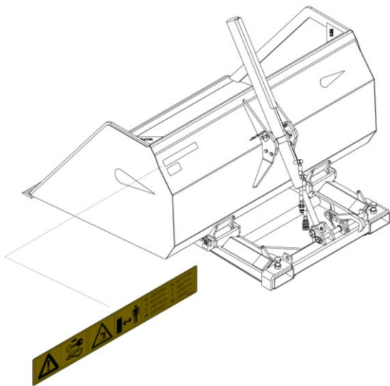
Abbildung 1.3.2-Stelle der Sicherheitsaufkleber für HO
