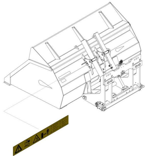
Abbildung 1.3.5 - Anbringungsstelle der Sicherheitsaufkleber für HO-ZIF
