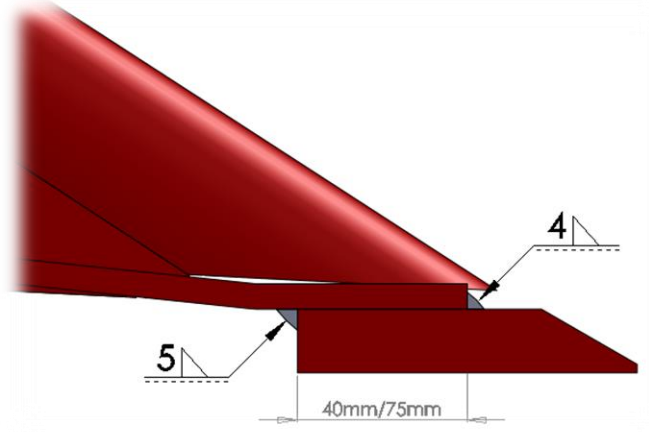
Figure 3.6.1 - Lame de recouvrement pour godet chargeur
