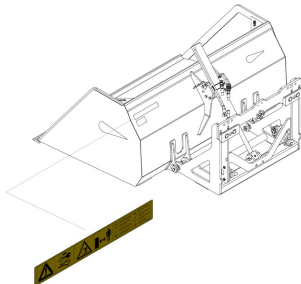
Abbildung 1.3.3-Position der Sicherheitsaufkleber für HO-F
