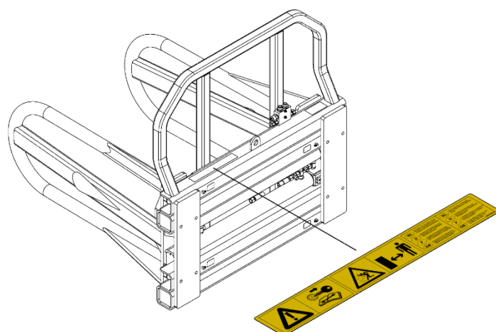
Figure 1.3.3-Modèle BKP-UF
