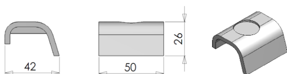
Figuur 14.2.6-MTT glijlager boven HS-2
