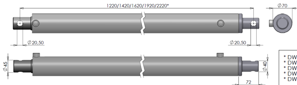
Figuur 8.1.2-Cilinder DW 60-50-1000/1200/1400/1700/2000
