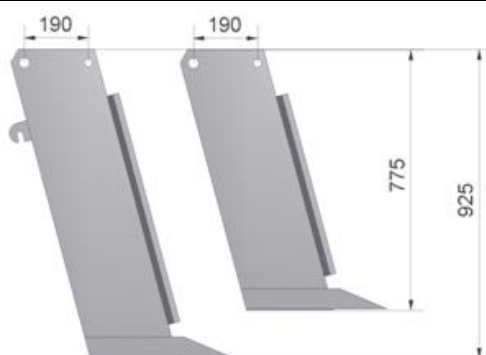
Figuur 17.1.12-Art.nr. 529014 (tand 775mm) Art.nr. 529015 (tand 925mm)
