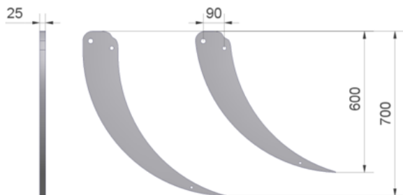
Figuur 6.3.9-Art.nr. 509035 (tand 600mm) Art.nr. 509036 (tand 700mm)
