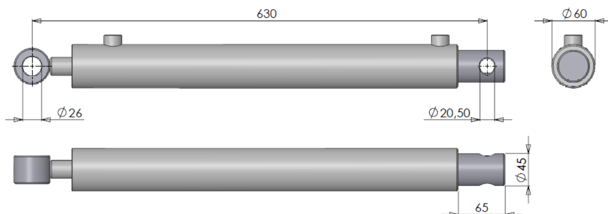
Figuur 3.1.2-Cilinder DW 50-25-410
