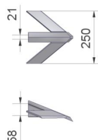
Figuur 17.1.8-Art.nr. 509525
