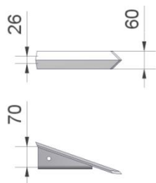
Figuur 6.3.12-Art.nr. 509054
