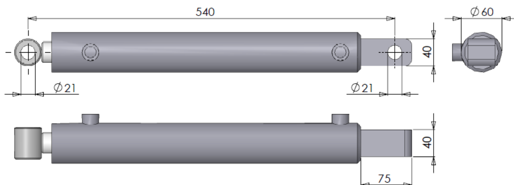
Figuur 3.1.4-Cilinder DW 50-30-330
