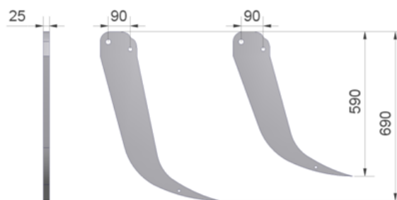
Figuur 17.1.2-Art.nr. 509037 (tand 590mm) Art.nr. 509038 (tand 690mm)
