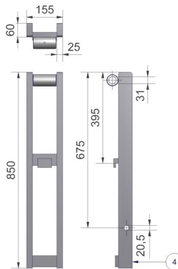
Figuur 8.2.4-Opstaande poot oud model met bus 1000-1600kg
