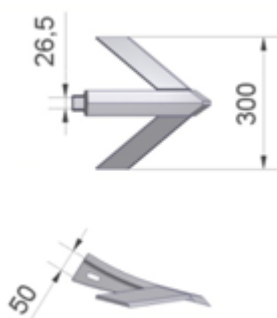
Figuur 6.3.15-Art.nr. 509067
