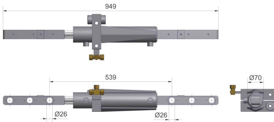
Figuur 3.1.6-Cilinder DW 60-30-250 (met T-koppeling)
