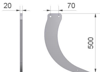
Figuur 17.1.5-Art.nr. 509506
