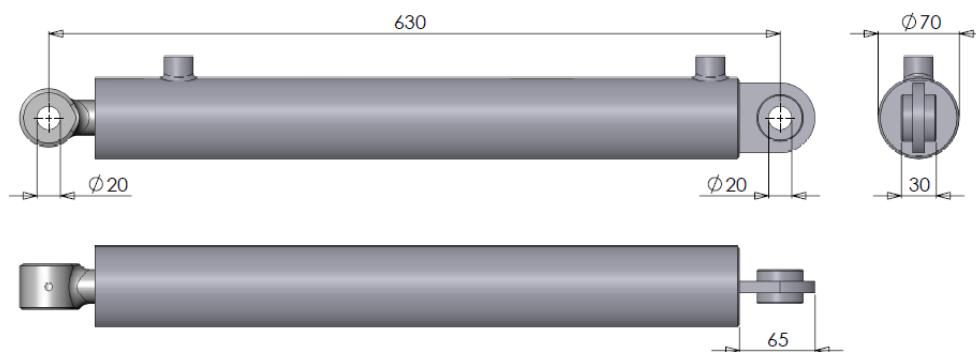
Figuur 2.1.2-Cilinder DW 60-30-410
