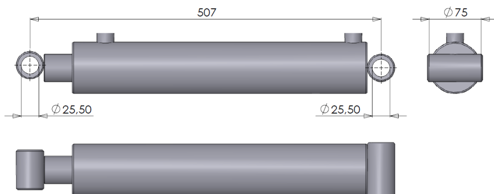
Figuur 10.1.1-Cilinder DW 63-40-320
