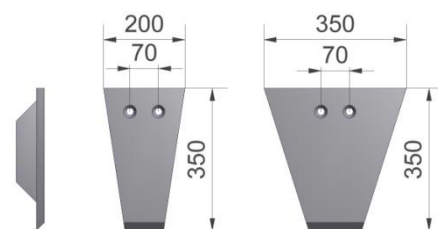
Figuur 17.1.14-Art.nr. 529032 (200mm) Art.nr. 529034 (350mm)
