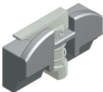
Figuur 13.1.3-Bovenklauw FEM II/III compleet
