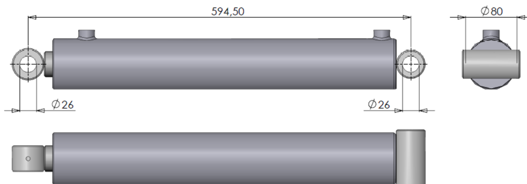
Figuur 3.1.12-Cilinder DW 70-40-410
