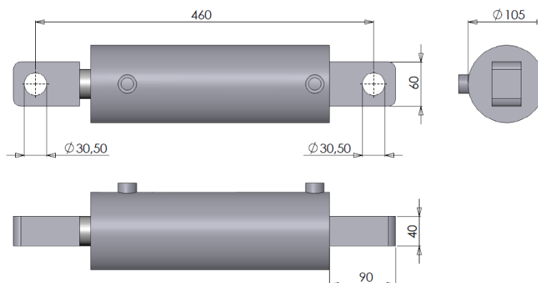
Figuur 3.1.15-Cilinder DW 90-40-200
