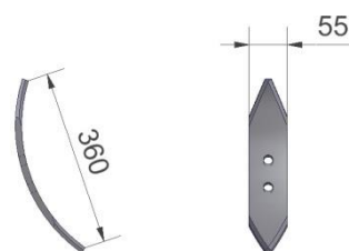
Figuur 6.3.21- 509051
