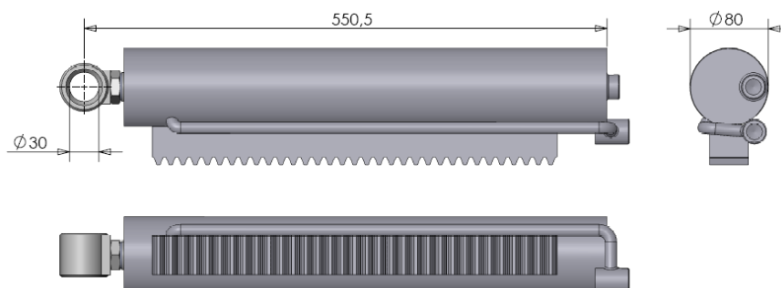
Figuur 3.1.11-Cilinder DW 70-30-377 (oud model)
