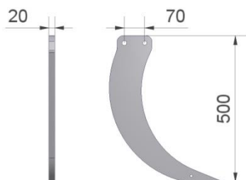
Figuur 6.3.3-Art.nr. 509506
