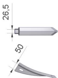
Figuur 17.1.3-Art.nr. 509053 Figuur 17.1.3-Art.nr. 509053A (Mangaan)
