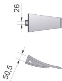
Figuur 17.1.5-Art.nr. 509055
