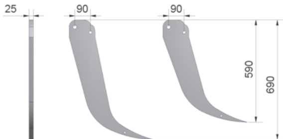
Figuur 6.3.10-Art.nr. 509037 (tand 590mm) Art.nr. 509038 (tand 690mm)
