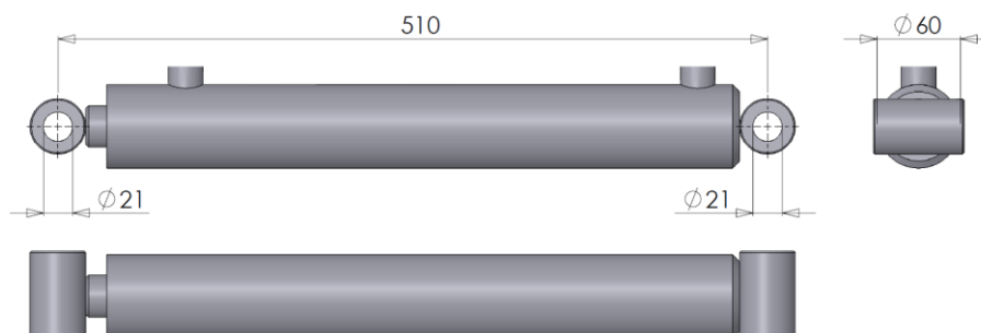
Figuur 12.1.1-Cilinder DW 50-30-330
