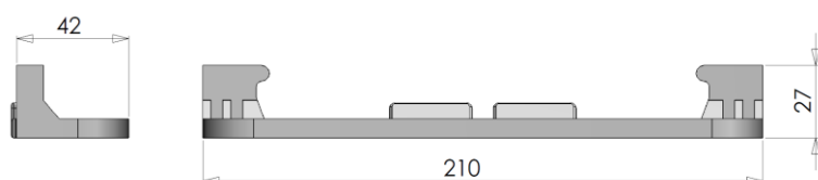
Figuur 14.2.2-CCD glijlager onder HS-2
