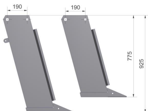
Figuur 17.1.16-Art.nr. 529009 (tand 775mm) Art.nr. 529010 (tand 925mm)
