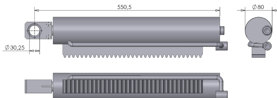
Figuur 3.1.10-Cilinder DW 70-30-377 (huidig model)
