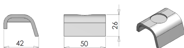
Figuur 14.2.6-MTT glijlager boven HS-2
