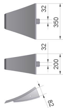
Figuur 17.1.21-Art.nr. 529031 (200mm) Art.nr. 529031A (200mm)(Mangaan) Art.nr. 529033 (350mm) Art.nr. 529033A (350mm)(Mangaan)
