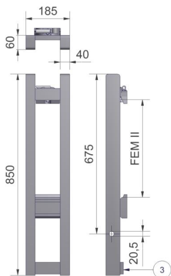
Figuur 8.2.3-Opstaande poot oud model FEM II 2000-2500kg
