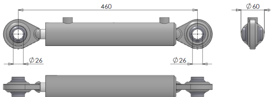
Figuur 8.1.4-Cilinder DW 50-25-200 cat. II-II
