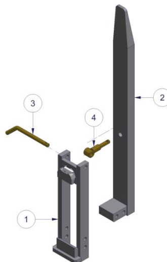
Figuur 13.1.2-Opklapbare lepel, model vanaf begin 2012
