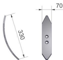
Figuur 6.3.8-Art.nr. 509052
