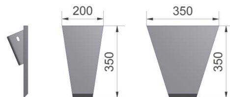
Figuur 17.1.18-Art.nr. 529027 (200mm) Art.nr. 529027A (200mm)(Mangaan) Art.nr. 529028 (350mm) Art.nr. 529028A (350mm)(Mangaan)
