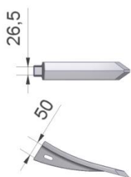
Figuur 6.3.11-Art.nr. 509053 Figuur 6.3.11-Art.nr. 509053A (Mangaan)
