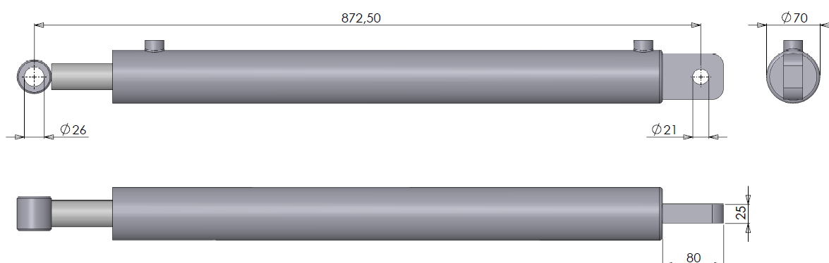
Figuur 14.1.3-Cilinder DW 60-35-600
