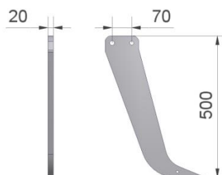
Figuur 6.3.4-Art.nr. 509509
