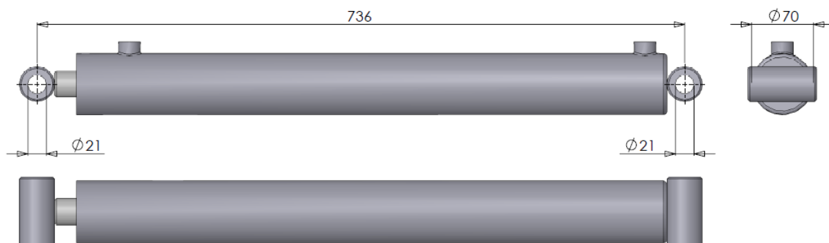
Figuur 3.1.7-Cilinder DW 60-35-550
