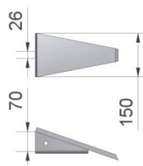
Figuur 17.1.6-Art.nr. 509056
