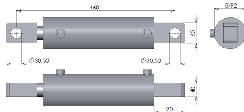
Figuur 3.1.14-Cilinder DW 80-40-200
