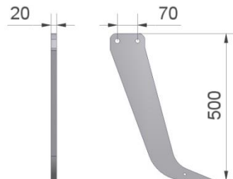
Figuur 17.1.6-Art.nr. 509509
