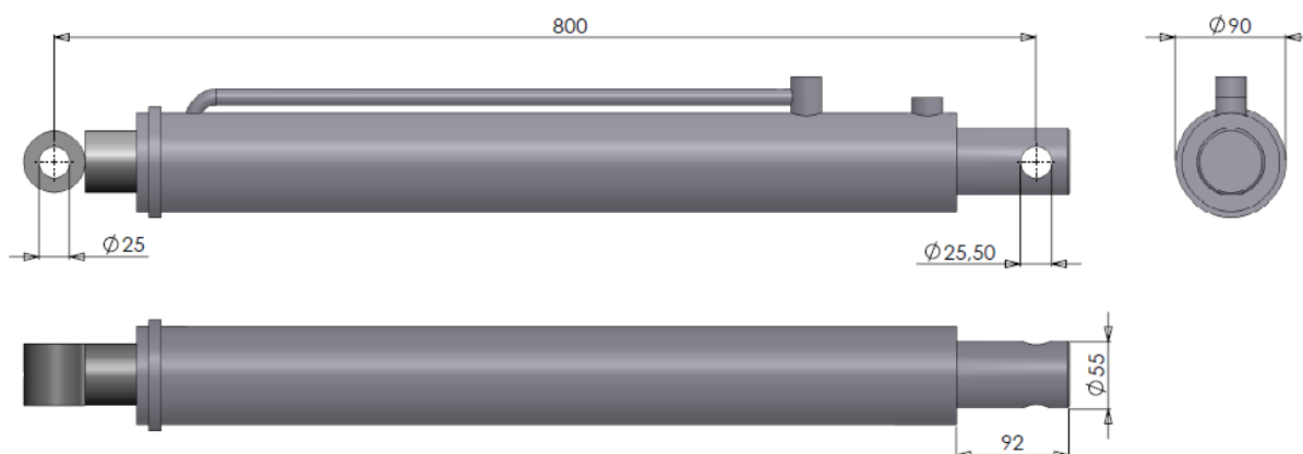
Figuur 3.1.13-Cilinder DW 70-50-550
