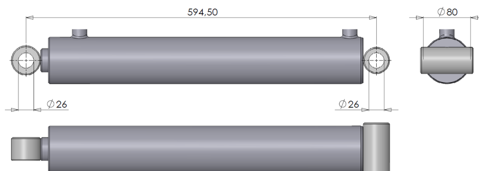
Figuur 12.1.3-Cilinder DW 70-40-410
