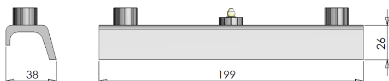
Figuur 14.2.3-CCD glijlager boven HS-3
