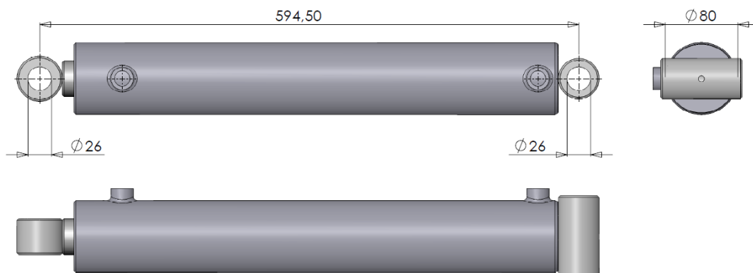
Figuur 10.1.2-Cilinder DW 70-40-410
