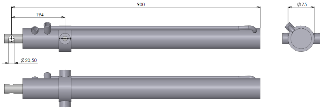
Figuur 9.1.1-Cilinder DW 63-35-750
