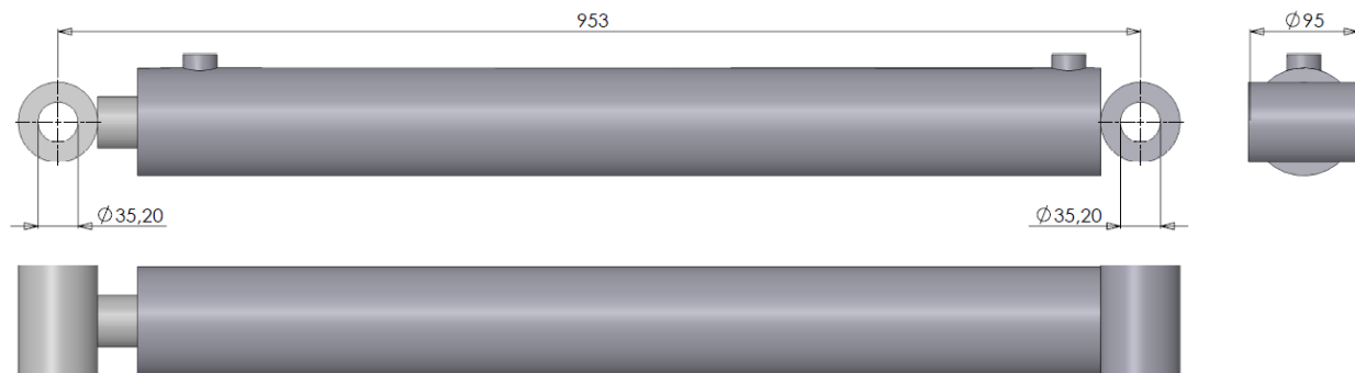
Figuur 6.1.2-Cilinder DW 80-45-700
