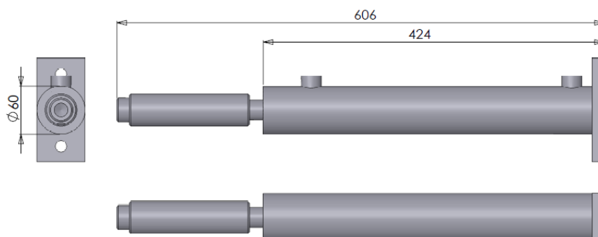
Figuur 14.1.2-Cilinder DW 50-25-300
