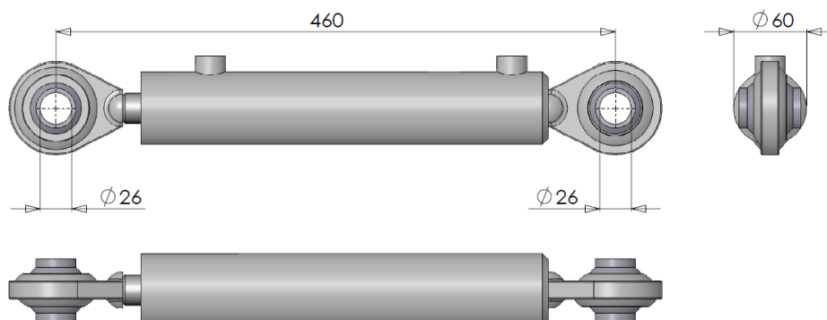
Figuur 3.1.1-Cilinder DW 50-25-200
