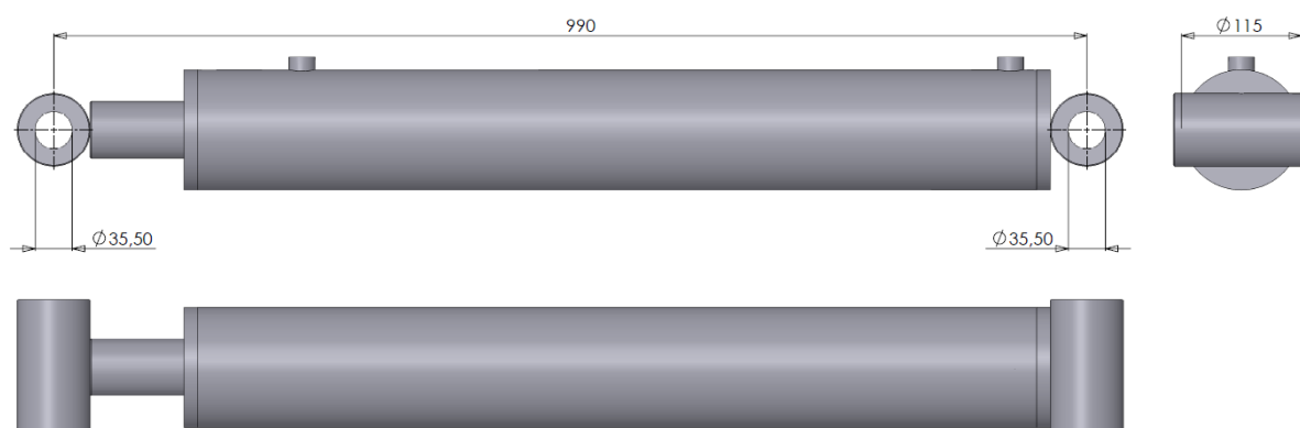
Figuur 5.1.4-Cilinder DW 100-55-670
