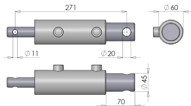
Figuur 7.1.1-Cilinder DW 50-25-50
