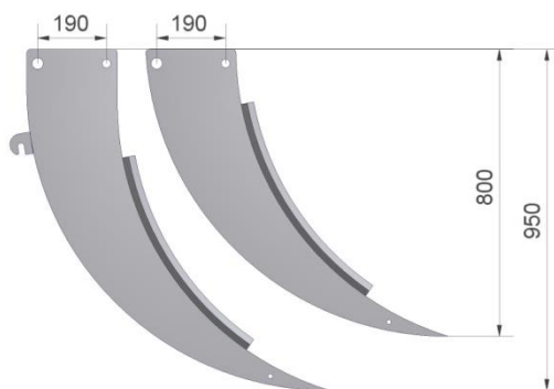
Figuur 17.1.19-Art.nr. 529011 (tand 800mm) Art.nr. 529012 (tand 950mm)
