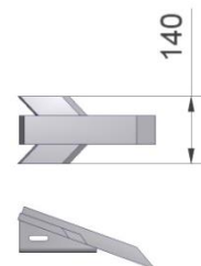
Figuur 17.1.11-Art.nr. 529030
