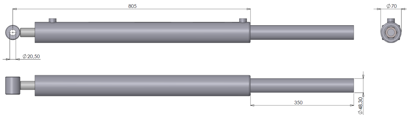
Figuur 5.1.1-Cilinder DW 60-30-600
