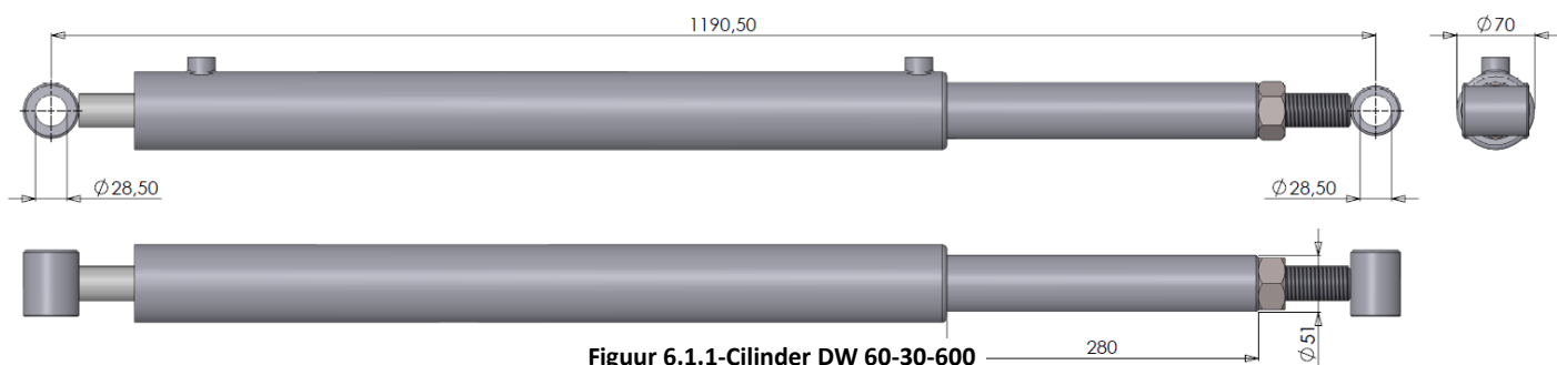
Figuur 6.1.1-Cilinder DW 60-30-600
