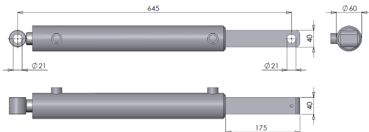
Figuur 3.1.3-Cilinder DW 50-30-330
