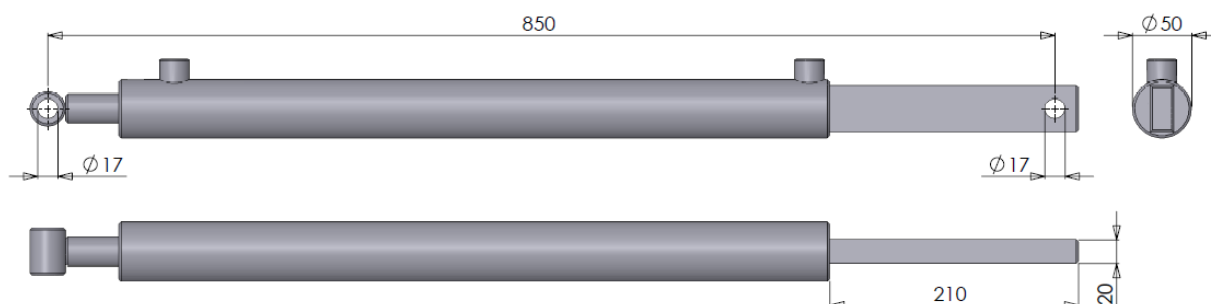
Figuur 14.1.1-Cilinder DW 40-25-500
