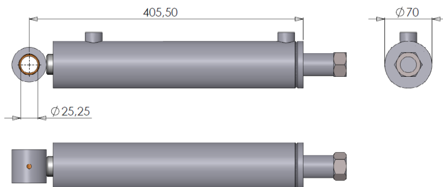
Figuur 3.1.5-Cilinder DW 60-30-250
