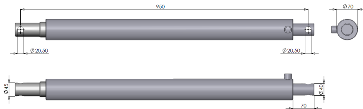
Figuur 2.1.1-Cilinder EW 50-700
