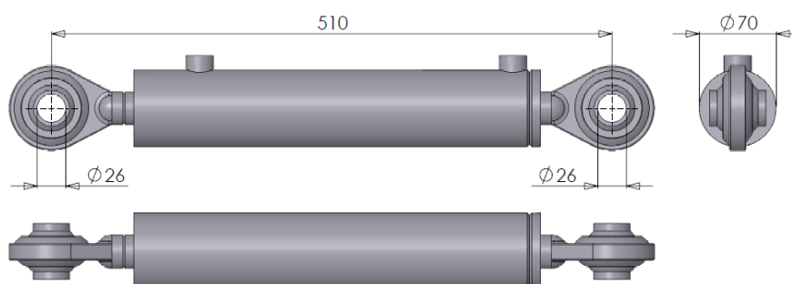
Figuur 12.1.2-Cilinder DW 60-30-250 cat. II-II
