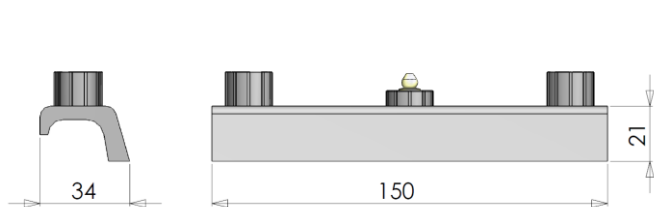
Figuur 14.2.1-CCD glijlager boven HS-2
