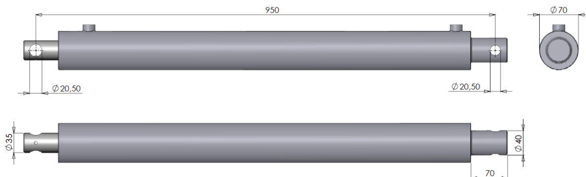
Figuur 2.1.3-Cilinder DW 60-35-700
