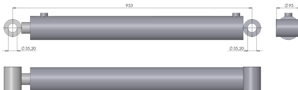
Figuur 5.1.3-Cilinder DW 80-45-700
