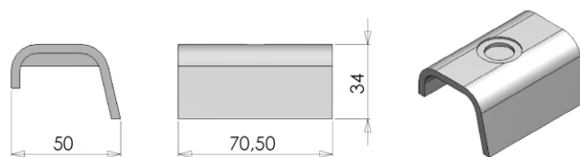
Figuur 14.2.7-MTT glijlager boven HS-3
