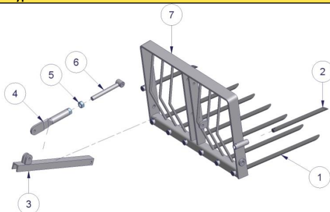
Type: Mestvork nr.3
