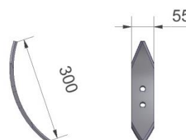
Figuur 6.3.2-Art.nr. 509522
