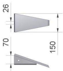
Figuur 6.3.14-Art.nr. 509056
