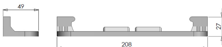
Figuur 14.2.4-CCD glijlager onder HS-3
