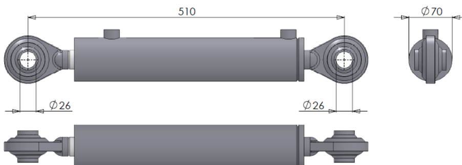
Figuur 8.1.5-Cilinder DW 60-30-250 cat. II-II
