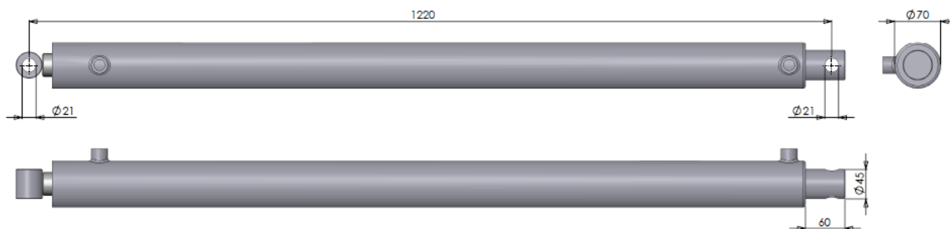
Figuur 3.1.9-Cilinder DW 60-35-1000
