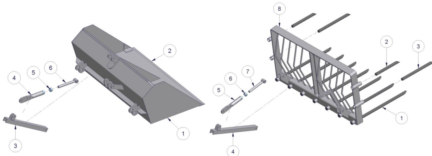
Type: Mestvork nr.3
