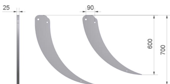
Figuur 17.1.1-Art.nr. 509035 (tand 600mm) Art.nr. 509036 (tand 700mm)
