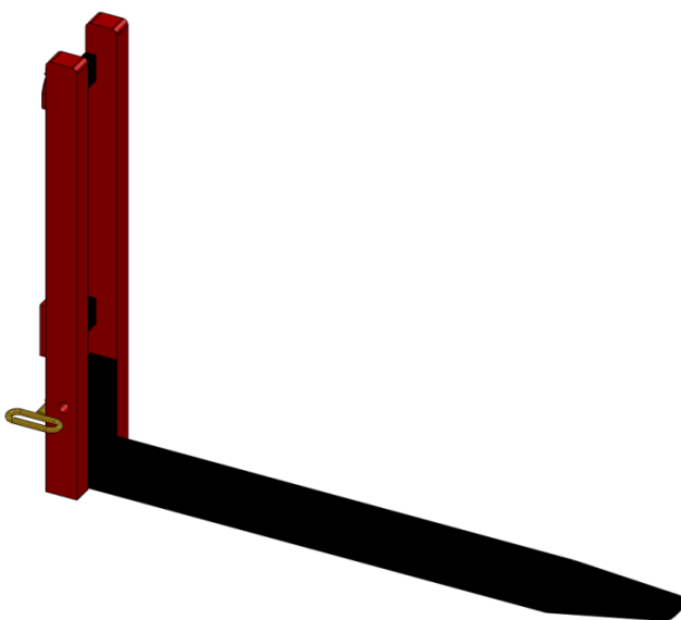
Figuur 2.4.5-Uitgeklapte lepel t.b.v. PF-25/PF-35
