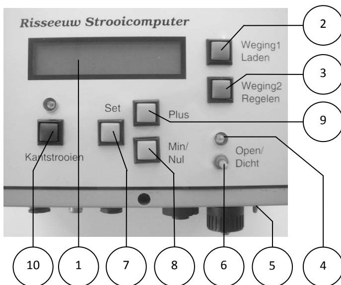
Figuur 3.2.3-Bedieningspaneel weeg-/strooicomputer
